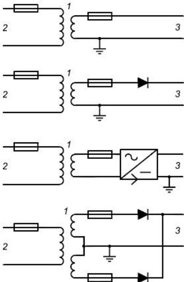
Рисунок 4 - Подача электроэнергии в цепь управления
