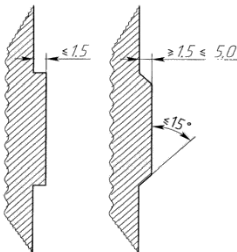
Рисунок 11 – Размеры допустимых выступов в зонах перемещения
