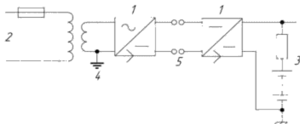
б) Зарядка аккумулятора постоянным током
