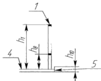
в) Вход на нижнюю посадочную площадку, предохранительная заслонка для платформ с перемещением до 500 мм
