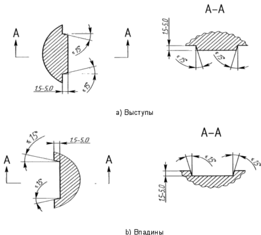
Рисунок 7 Скосы краев и впадин
