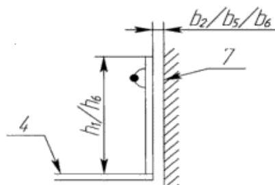
г) Ограничение доступа к краям платформы; предохранительный неперфорированный барьер для платформ с перемещением более 2000 мм, использование барьера в качестве поручня
