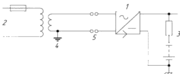
а) Зарядка аккумулятора переменным током
