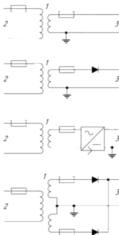
1 – разделительный трансформатор; 2 – первичный источник электроэнергии; 3 – цепь управления
